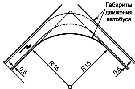
Рисунок Г.1 - Пример построения закругления с отгонами уширения и с единой круговой кривой
