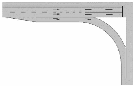
г) Полоса для поворота с направляющим островком с полосой разгона
