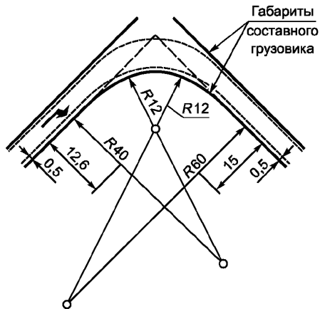
Рисунок Г.2 - Пример построения закругления с серией круговых кривых из трех частей
