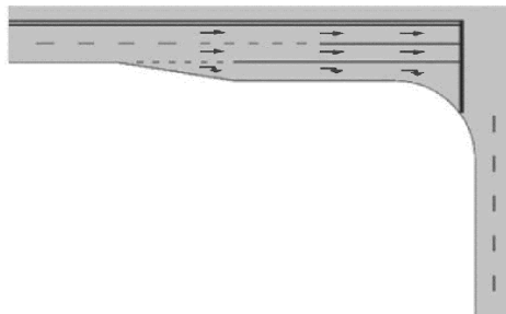
б) Полоса для поворота без направляющего островка
