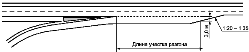
б) Параллельная полоса разгона
