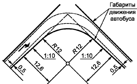
Рисунок Г.1 - Пример построения закругления с отгонами уширения и с единой круговой кривой
