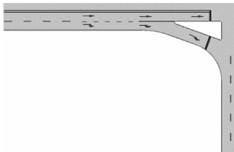
в) Полоса для поворота с направляющим островком без полосы разгона
