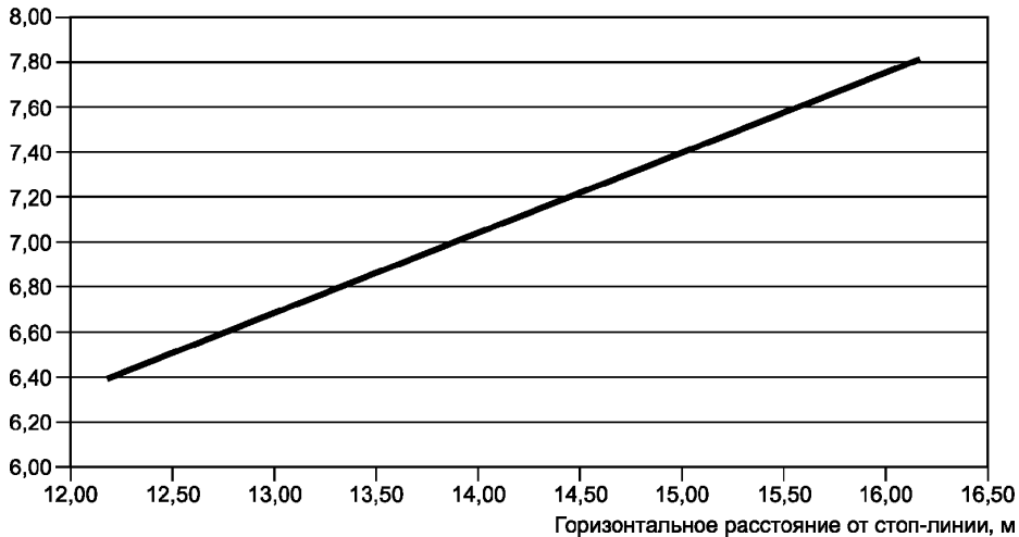
Рисунок Д.2 - Максимальная высота установки верхнего сигнала светофора над проезжей частью
