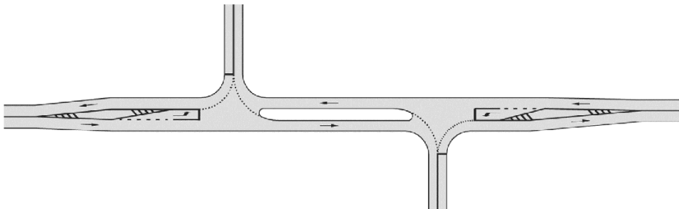
а) Левое смещенное пересечение
