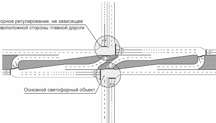
Рисунок 19 - Пересечение в одном уровне с отнесенными левыми поворотами с второстепенной дороги и левым поворотом с главной дороги без обеспечения прямого проезда
