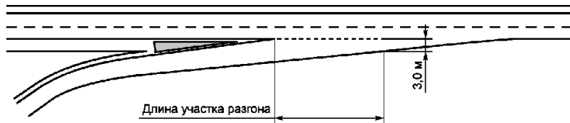
а) Диагональная полоса разгона
