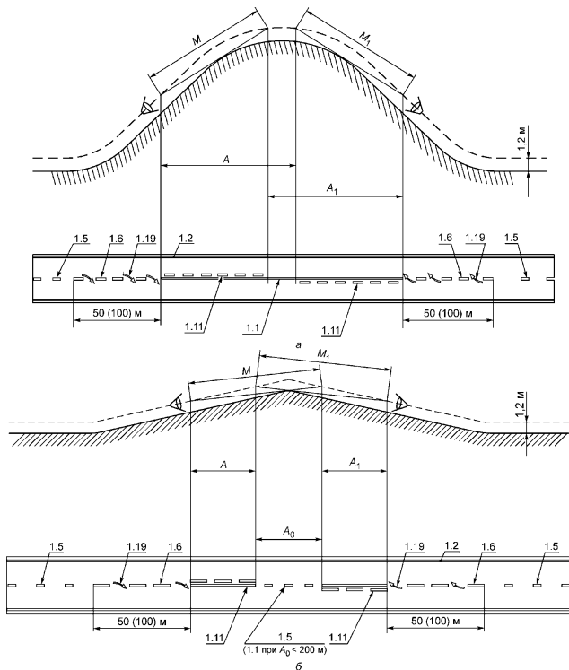
Рисунок В.5 - Пример расстановки знаков 5.1 и 5.2
