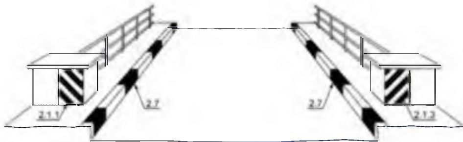
Рисунок В.23 - Пример нанесения разметки 2.1.1, 2.1.3 и 2.7
