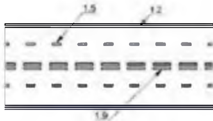
Рисунок В.17 - Примеры нанесения разметки 1.9
