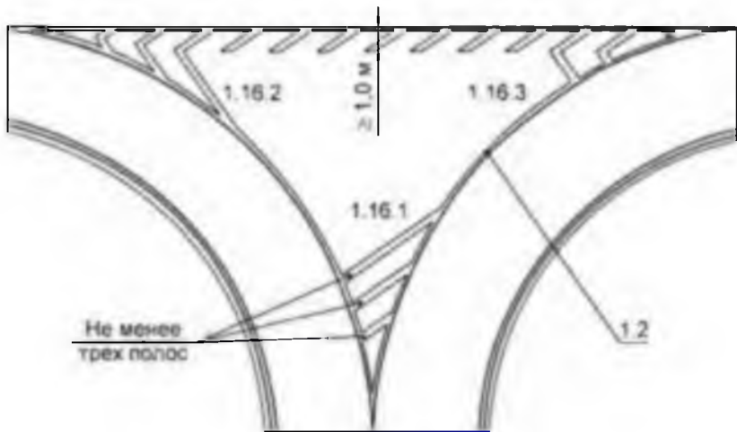
Рисунок В.12 - Пример нанесения разметки 1.16.1 - 1.16.3
